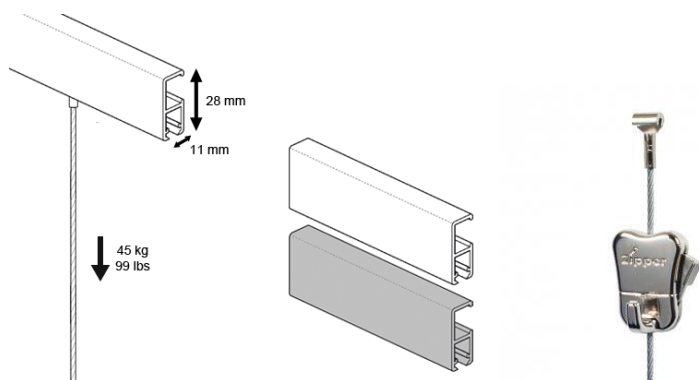
Σχέδιο ραγών αλουμινίου και συρματόσχοινου
