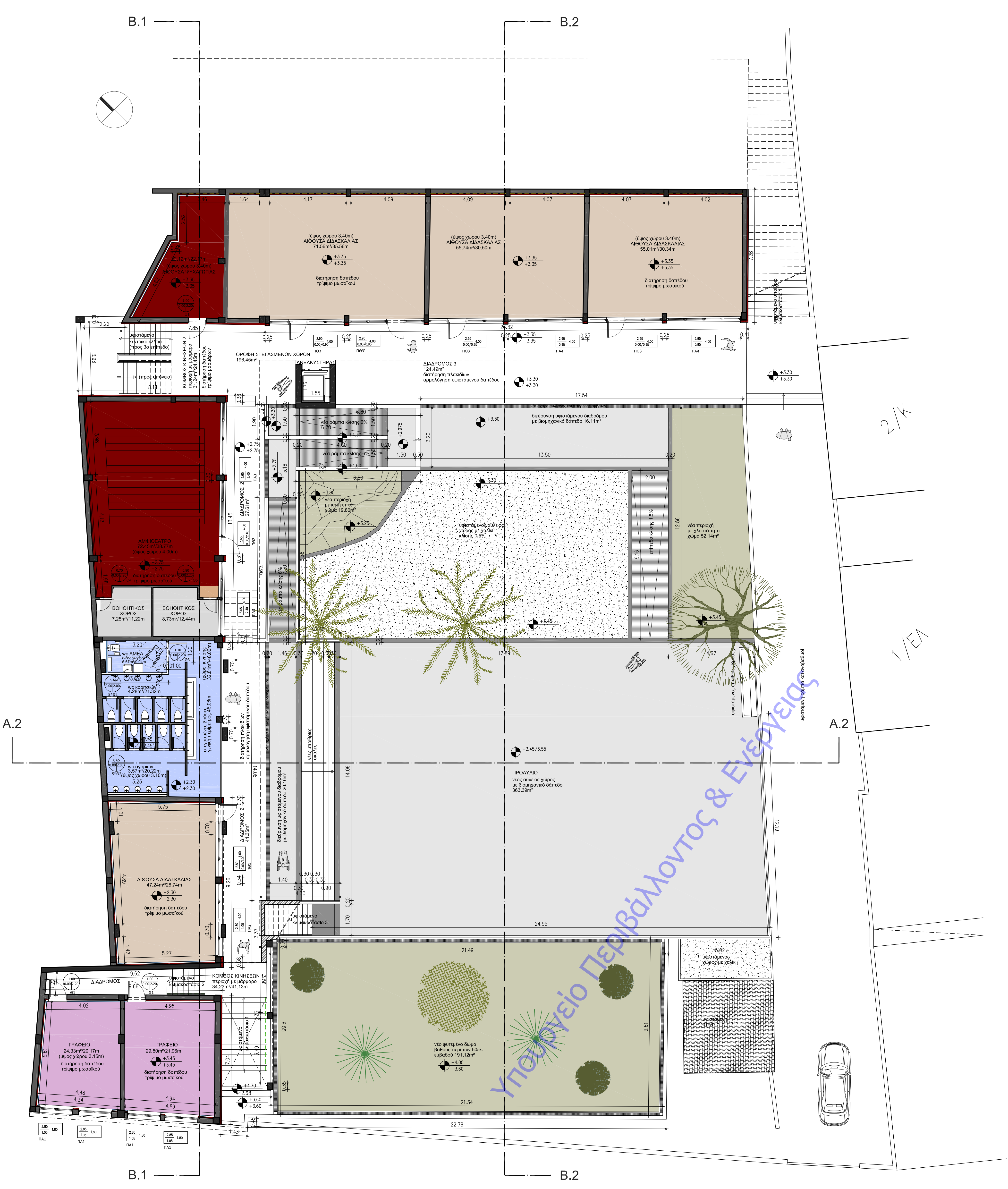
ΚΑΤΩΦΗ 2ου ΕΠΙΠΕΔΟΥ ΓΥΜΝΑΣΙΟΥ ΝΕΑΠΟΛΗΣ Α' ΟΡΟΦΟΣ & ΙΣΟΓΕΙΑ ΚΤΙΡΙΟΥ ΤΟΥ ΠΡΟΑΥΛΙΟΥ ΧΩΡΟΥ
